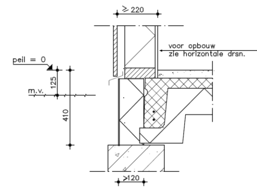
detail 6 –vliesgevel
