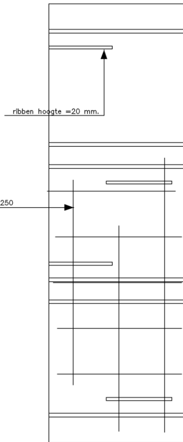
isolatiedoos type 2400
