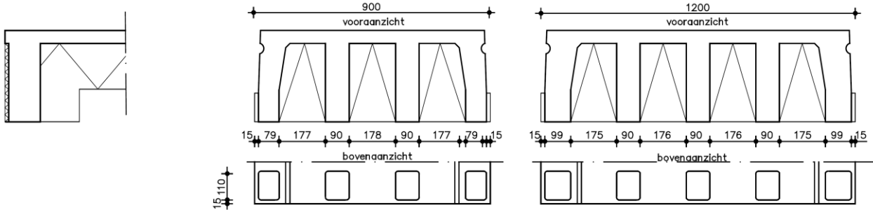
gesoleerd kopschot met oplegnokken
