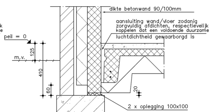
betondetail 5
