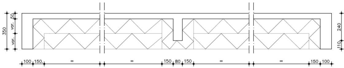
langsdoorsnede type 2400 met dwarsrib
