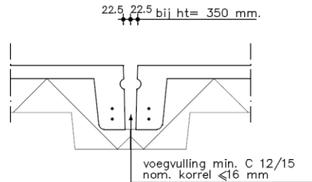
voegdetail
